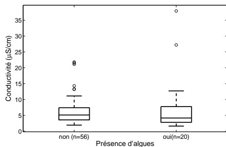
FIG. 3.23 – Conductivité électrique constatée en l'absence et en présence d'algues de neige.
